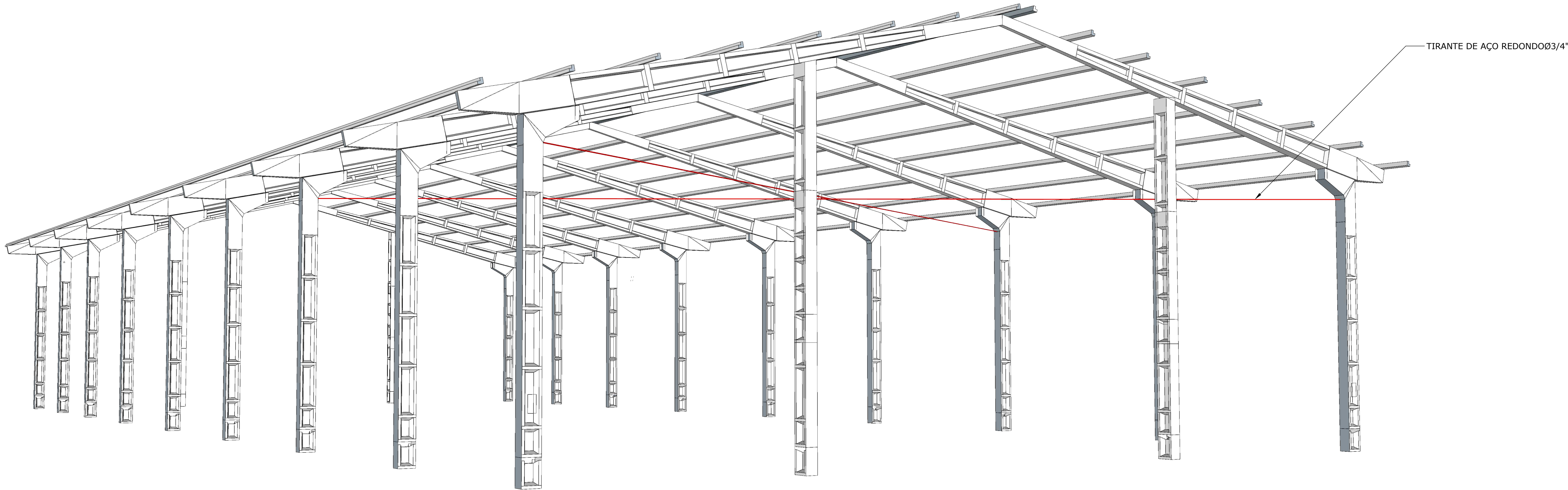
PERSPECTIVA ESTRUTURA Sem escala
